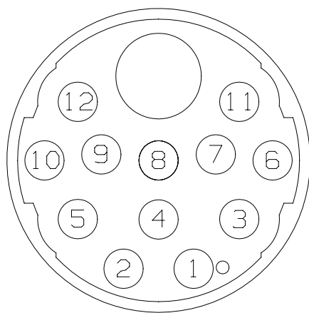
SOLDER LUG VIEW
